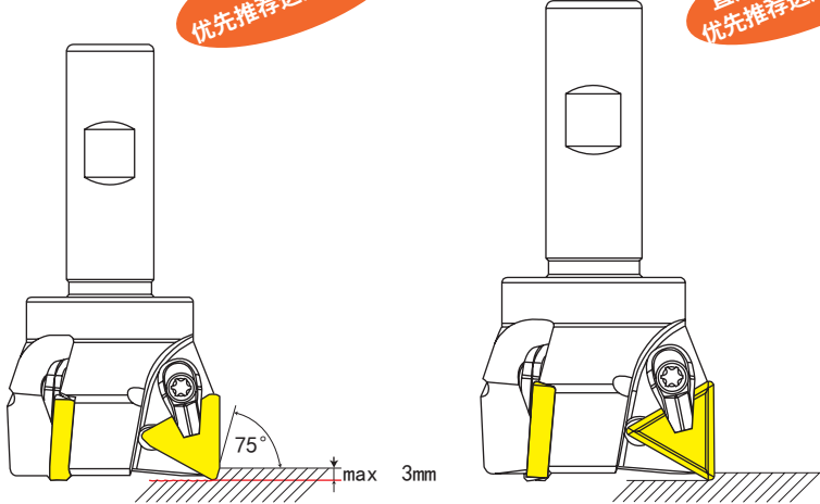
XPKN 220412 钢用 材质 PP30
