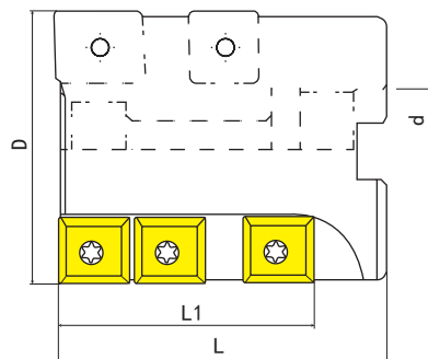
槽、切入加工 Slot, plunge milling
