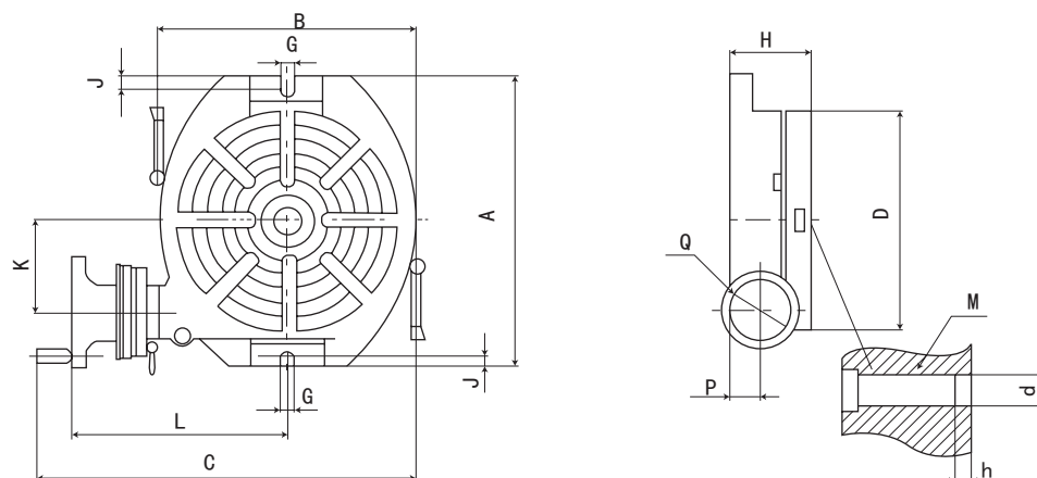
TS...A 系列回转工作台安装尺寸图 DIMENSIONAL SKETCH
