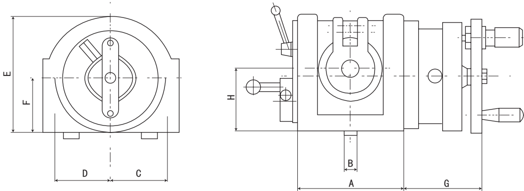
F12 系列半万能分度头安装尺寸参数: Installation sketch and dimensions
